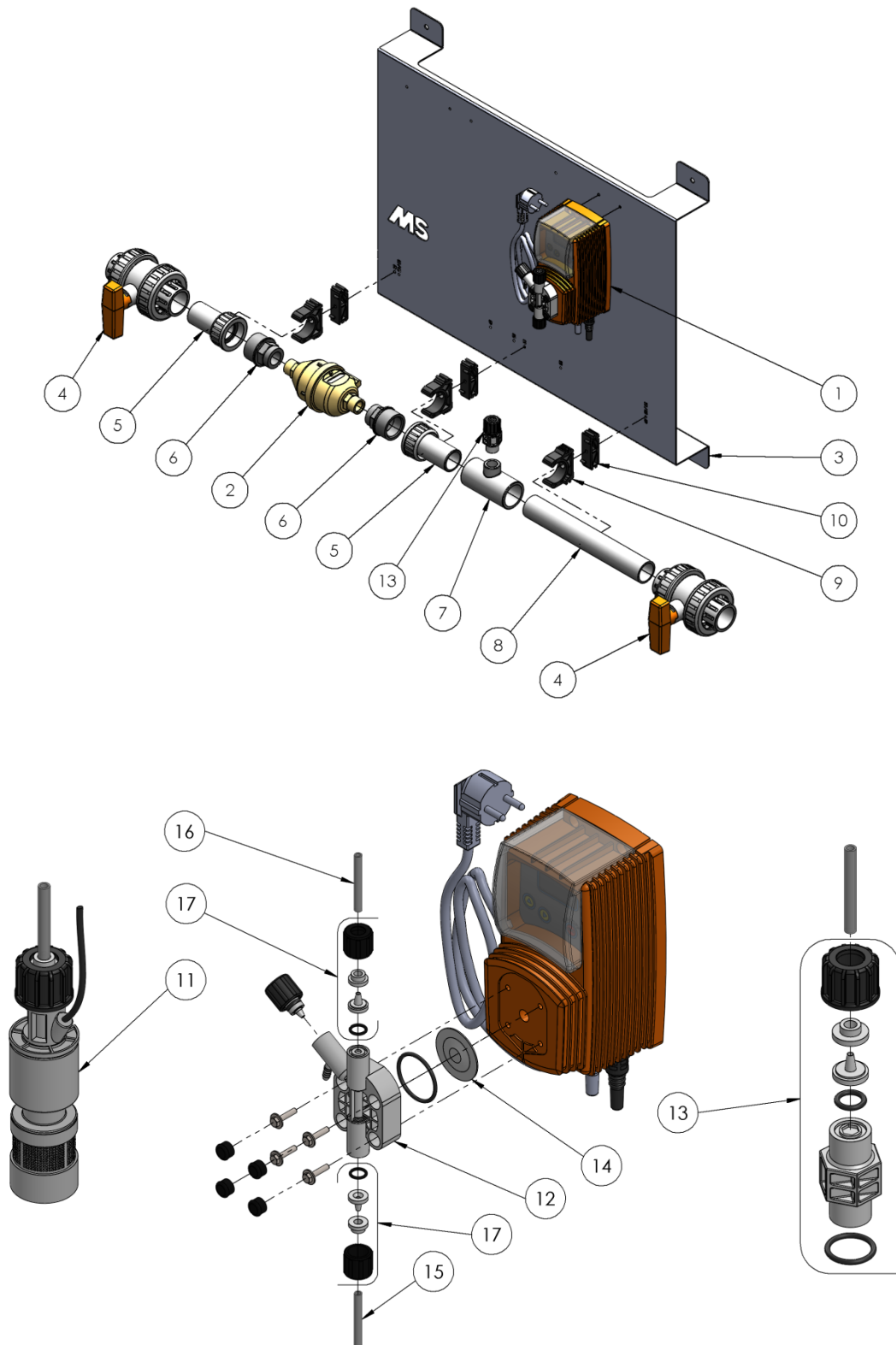
Abb. 1.1 Explosionszeichnung
